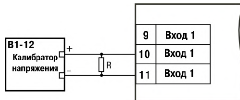
Рисунок 11.4 – Подключение калибратора напряжения 2
