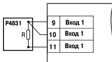
Рисунок 11.2 – Схема соединения с магазином сопротивлений
