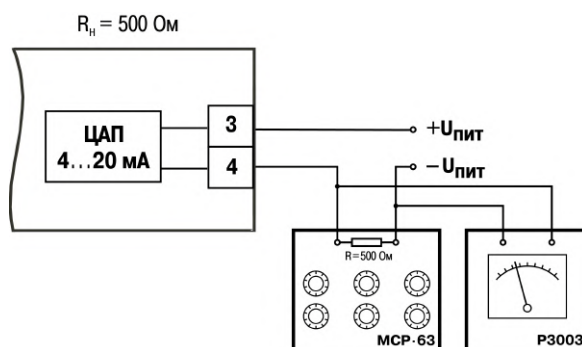
Рисунок 11.5 – Схема подключения к ВЭ типа «И»
