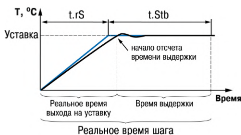
Рисунок 7.6 – Пример условий перехода
