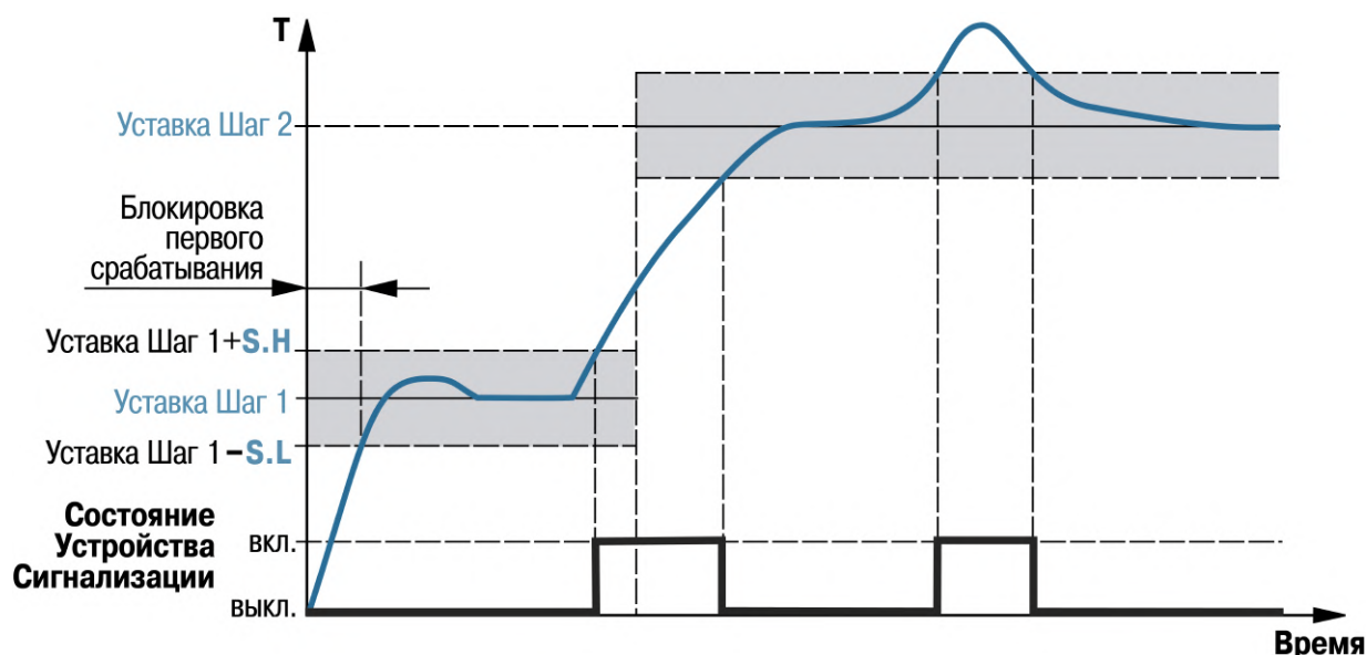
Рисунок 10.22 – Пример логики работы и блокировки срабатывания устройства сигнализации для U-образной логике
