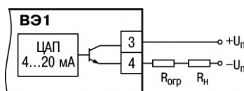
Рисунок 5.13 – Схема с ограничительным резистором
