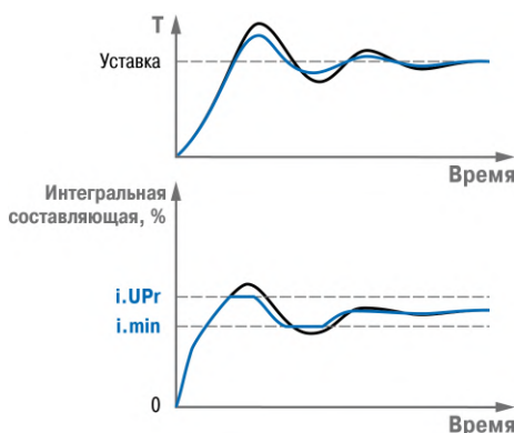
Рисунок 7.8 – Пример ПИД-регулирования
