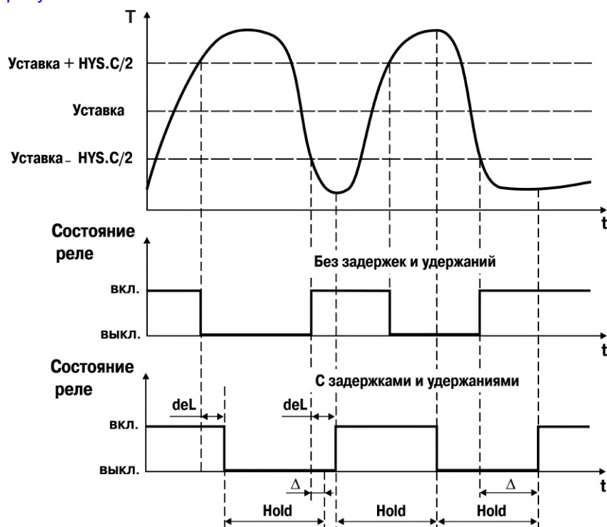
Рисунок 10.17 – Работа регулятора с заданным удержанием
