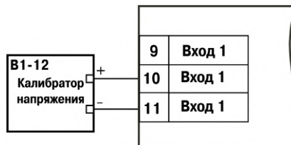
Рисунок 11.3 – Подключение калибратора напряжений
