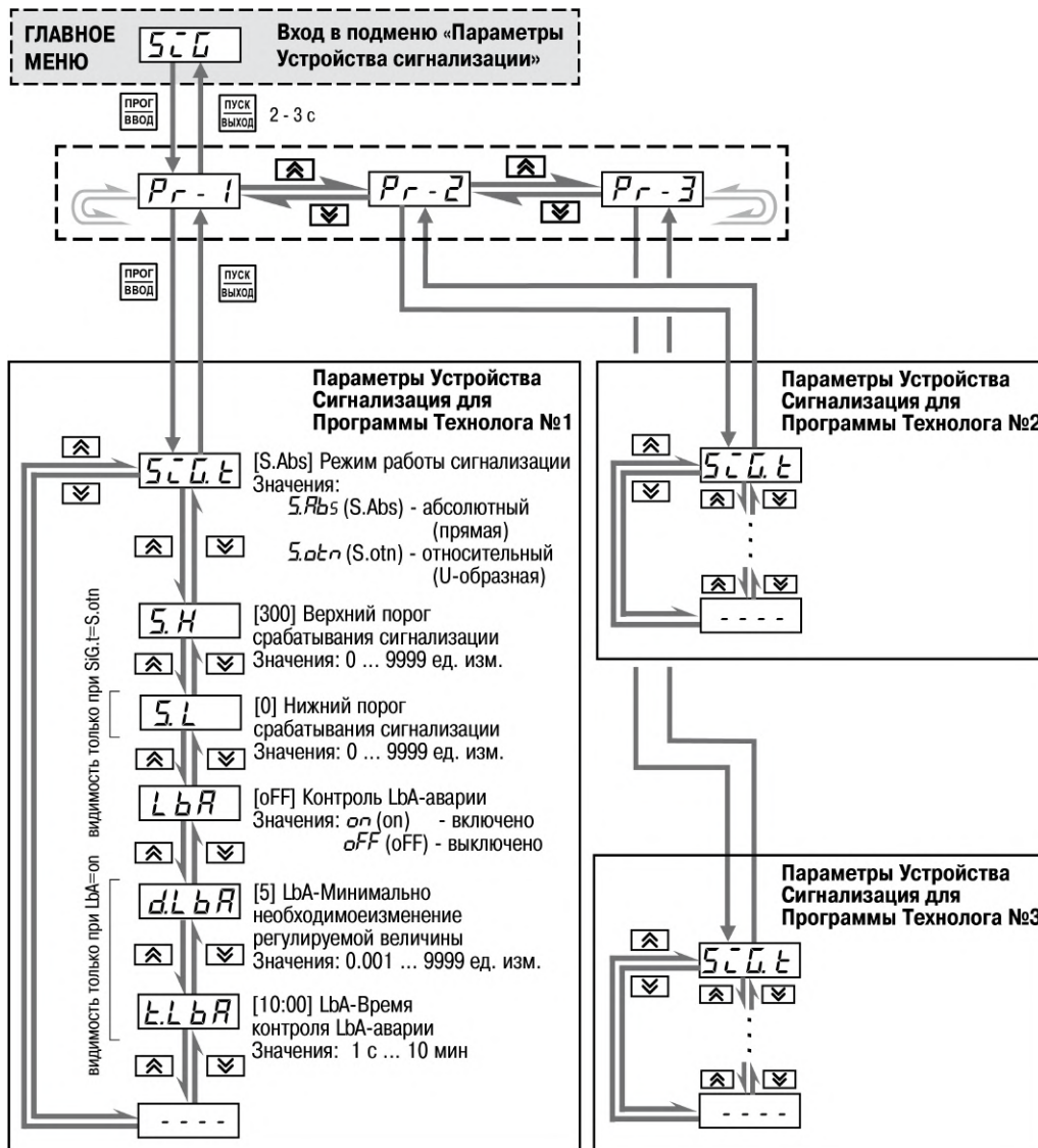
Рисунок 8.4 – Параметры устройства сигнализации
